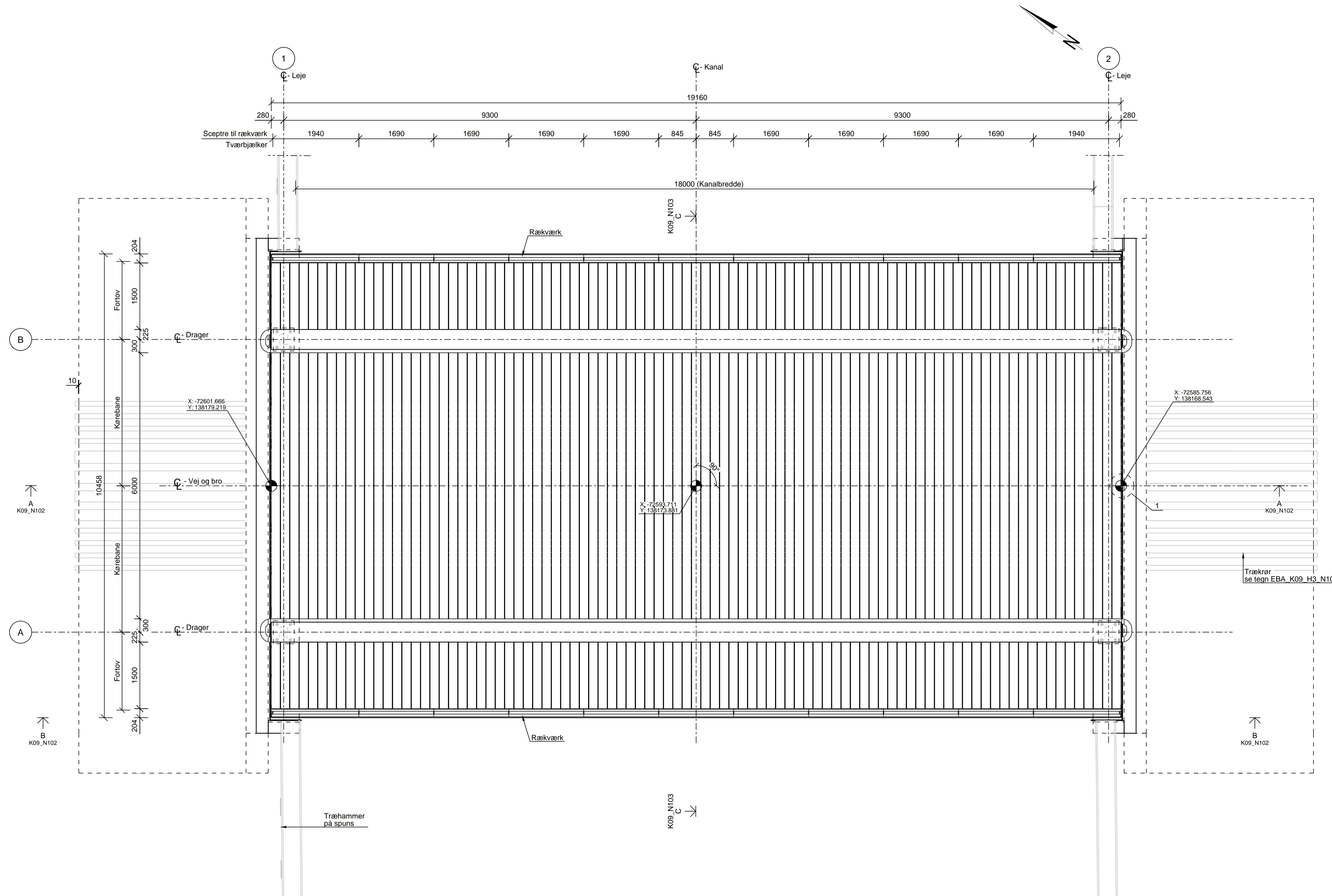
PLAN, 1:50
