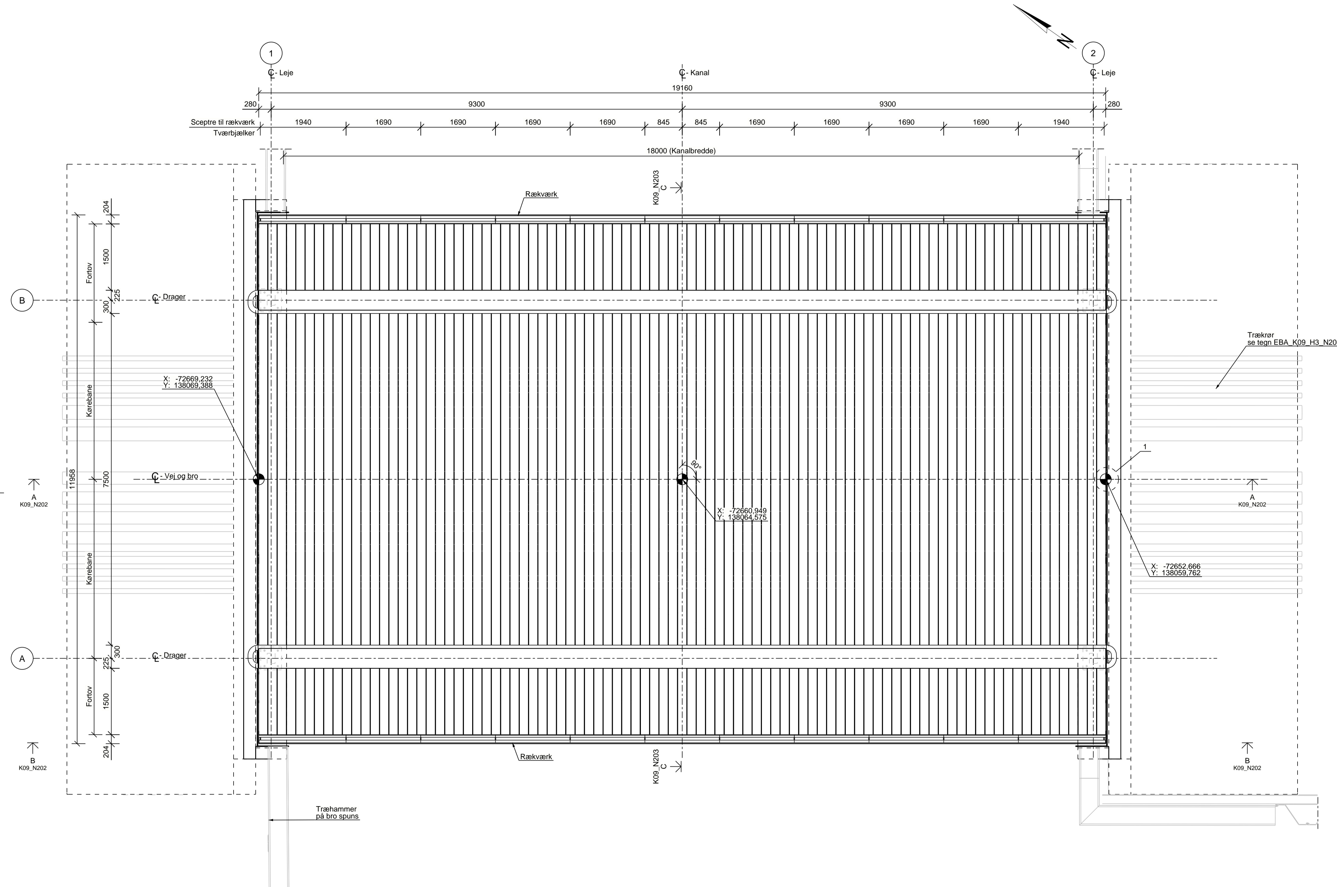
PLAN, 1:50
