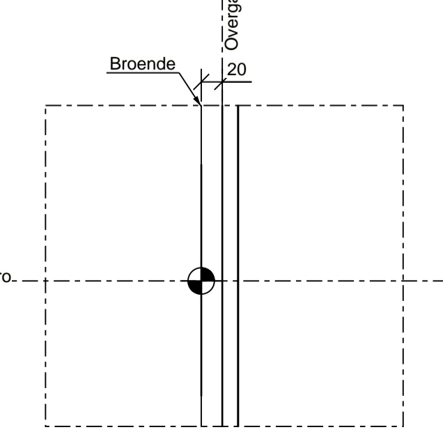
DETALJE 1, 1:5
