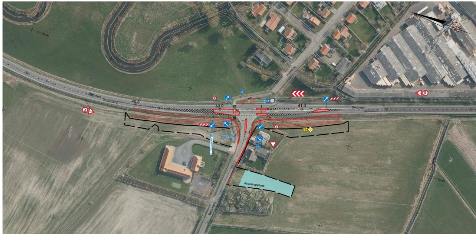
Bjerrumvej og Rute 11 ved Ribe med ombygningen skitseret
