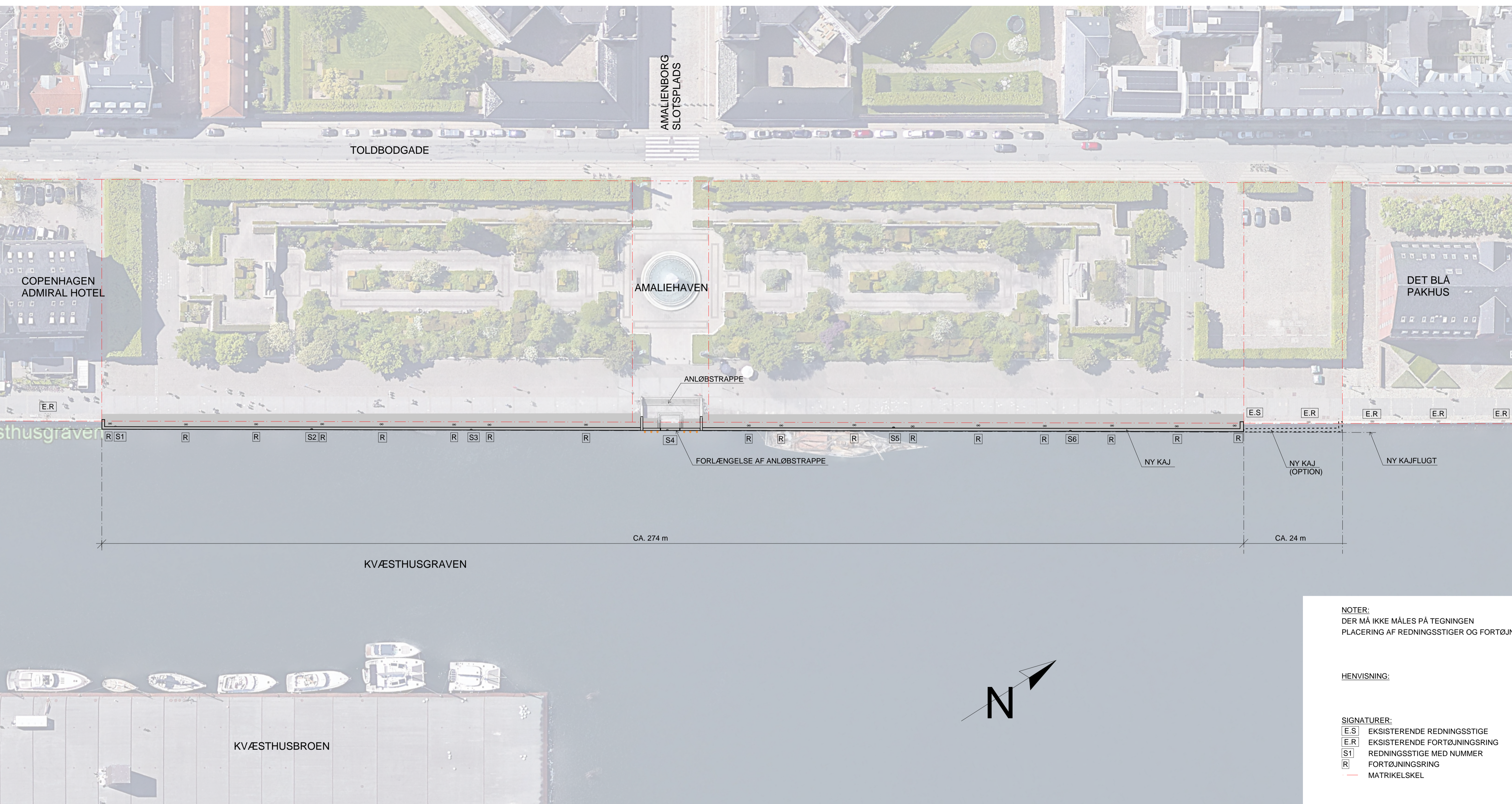
OVERSIGTSPLAN, 1:500
