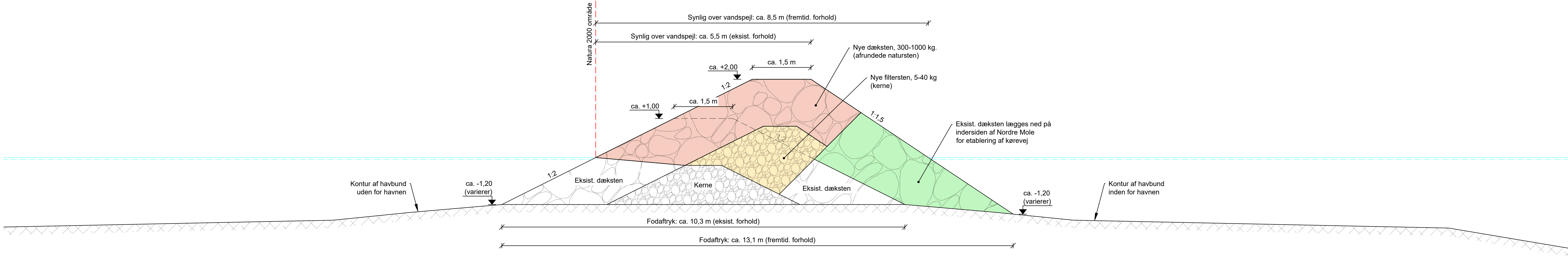
Tværsnit A, 1:50
