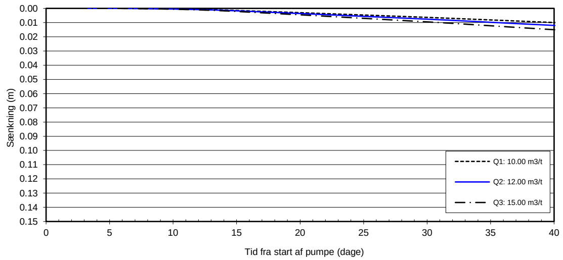
Sænkningsskurver, 100 m
