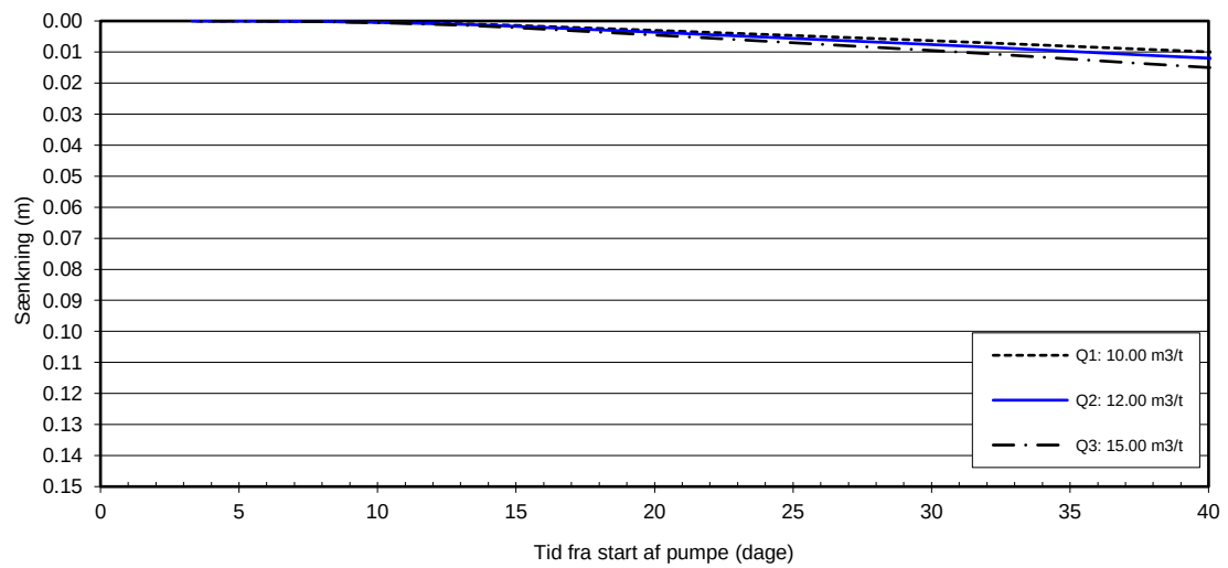
Sænkningsskurver, 250 m
