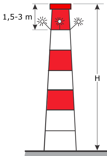
Figur 2-2: Afmærkning af skorstene
