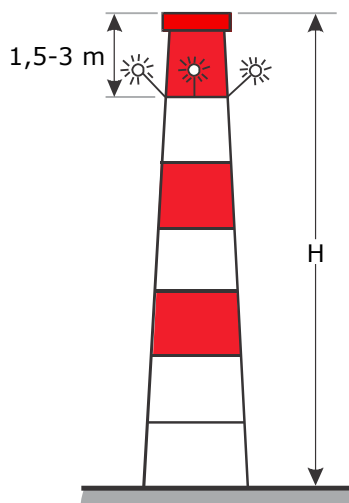
Figur 18-2: Afmærkning af skorstene
