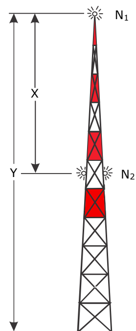
Figur 18-1: Dagafmærkning og placering af hindringslys. Y er højden over terræn eller omkringliggende terræn, og X er den maksimale afstand jf. pkt. 10.12, 10.15, 10.16 og 10.18.
