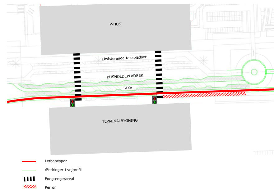
Figur 14. Billund Lufthavn forplads, Vejle-løsning (letbane)
