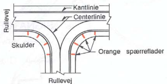
Spærreflade for luftfartøjer. Orange farve. Afmærkningen benyttes for at fremhæve ikke bæredygtig skulderbelægning i rullevejskryds og i rullevejssving og steder, hvor det er vanskeligt at skelne kantafmærkningen fra rullevejscenterlinien. Afmærkning anvendes også på manøvreområdet.
