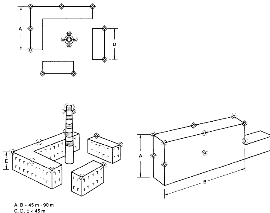
Figur 6-4 Afmærkning på bygninger
