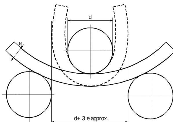
Tegning af bøjepróve (approx. = ca.)
