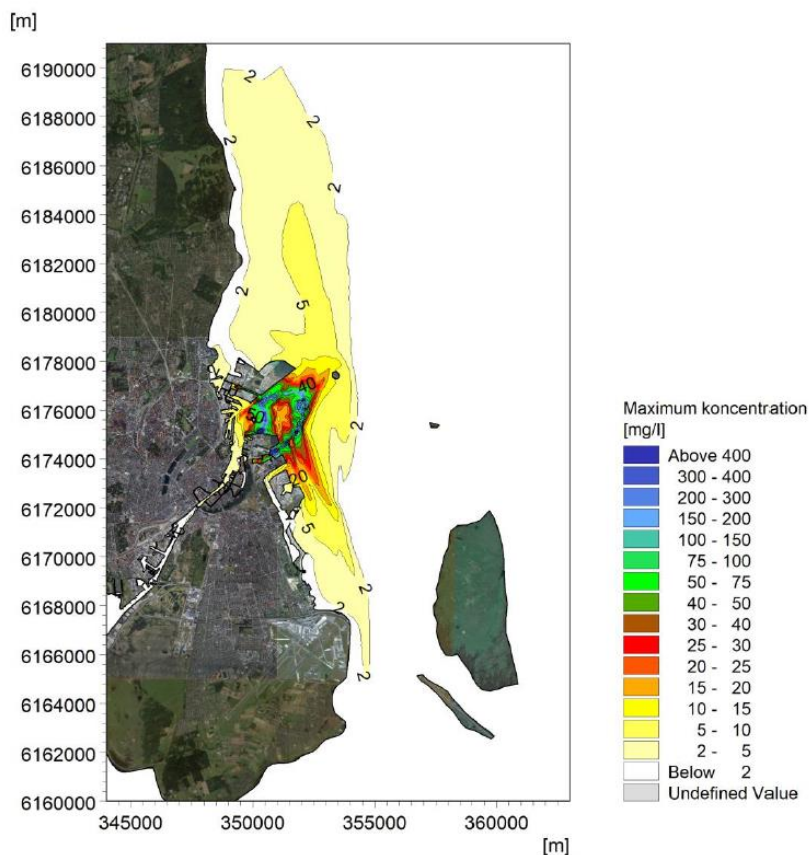
Figur 4-10: Modelleret dybdemidlet maksimum sedimentkoncentration udløst af gravespild.
