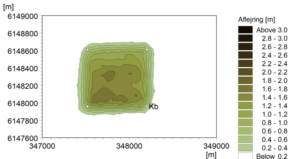
Figur 5-21 Aflejringsstykkelse på klappads Kb efter klapping i perioden oktober 2021 – marts 2022.
