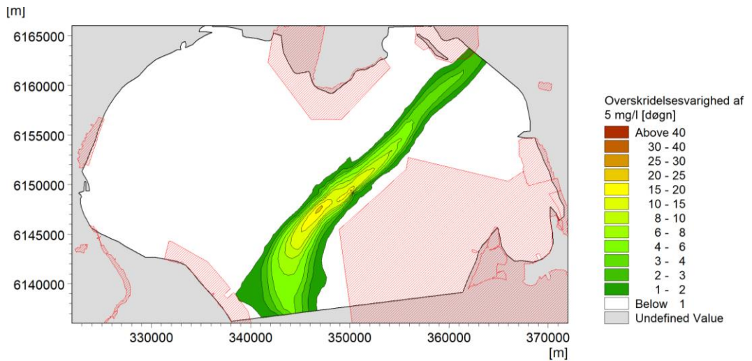
Figur 5-30 Overskridelsesvarighed af 5 mg/l i vinterhalvåret (oktober-marts) med klapping på Ka og Kb.
