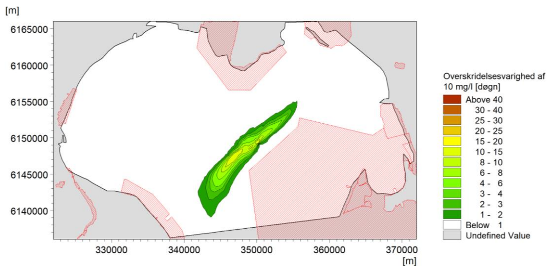
Figur 5-31 Overskridelsesvarighed af 10 mg/l i vinterhalvåret (oktober-marts) med klapping på Ka og Kb.
