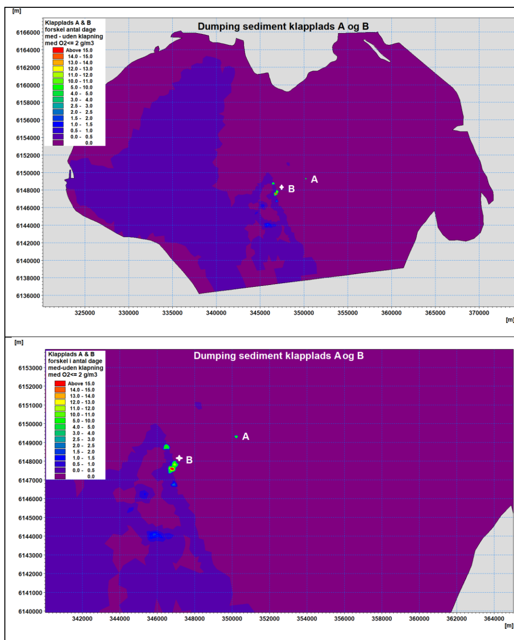
Figur 7-6 Ændring (førøgelsen) i antal dage med beregnede ilt koncentrationer under 2 mg/l i bundlaget. Klappning på plads A og B, (øverst hele området, nederst et zoom omkring klappbladsene).
