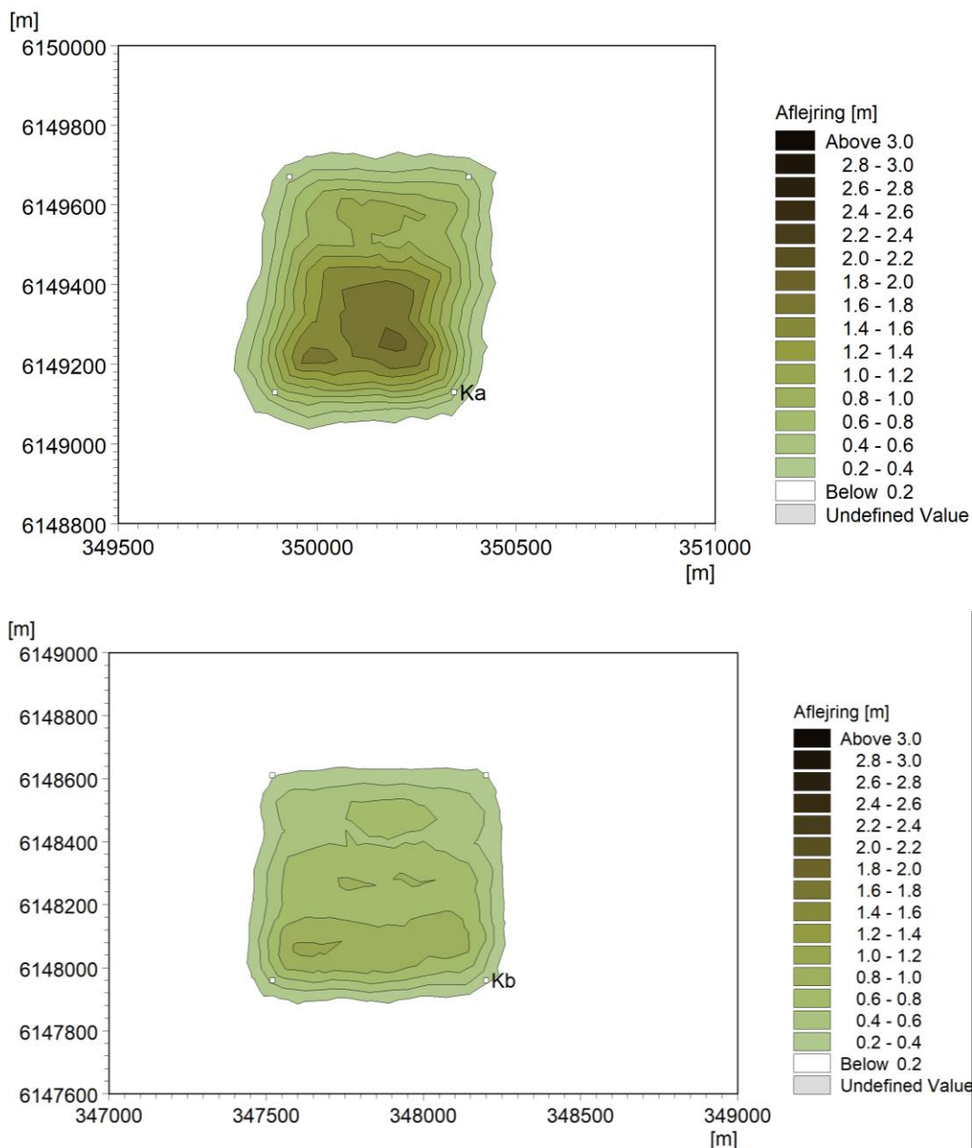
Figur 5-33 Aflejringstykkelse på klappplads Ka og Kb efter klapping i perioden oktober 2021 – marts 2022.
