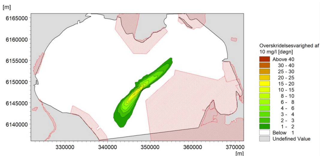
Figur 5-18 Overskridelsesvarighed af 10 mg/l i vinterhalvåret (oktober-marts) med klapping på Kb.
