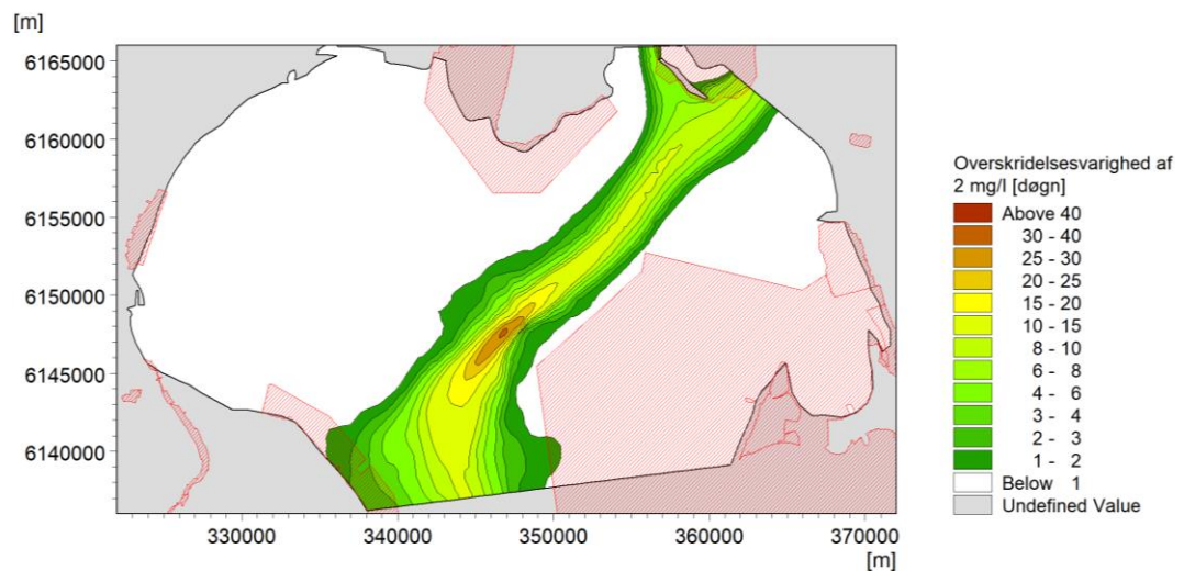
Figur 5-16 Overskridelsesvarighed af 2 mg/l i vinterhalvåret (oktober-marts) med klapping på Kb.
